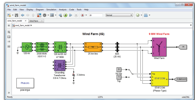
Obr. 2 Ilustrační model energetické soustavy v prostředí Simulink
